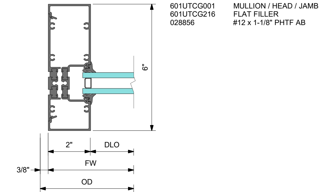
4 DETAIL 4 JAMB
