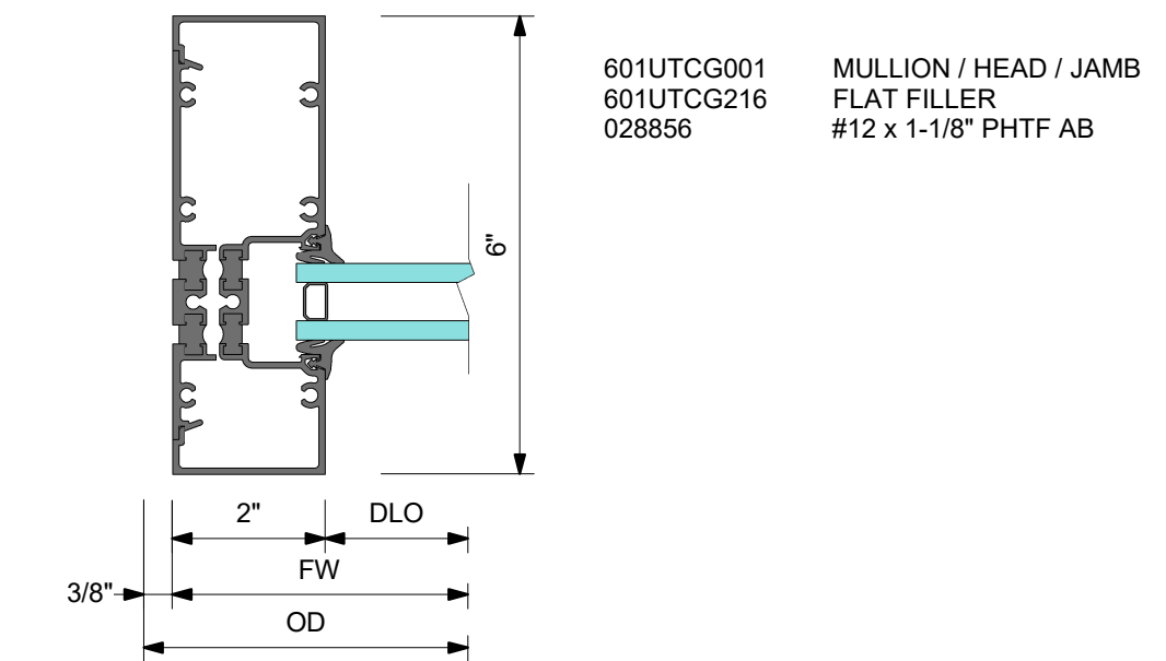
4 DETAIL 4 JAMB
