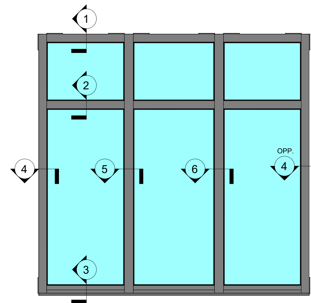
ELEVATION
