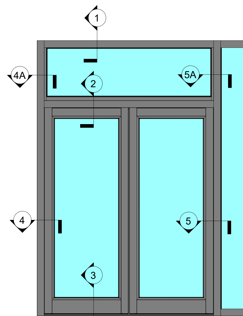
ELEVATION
