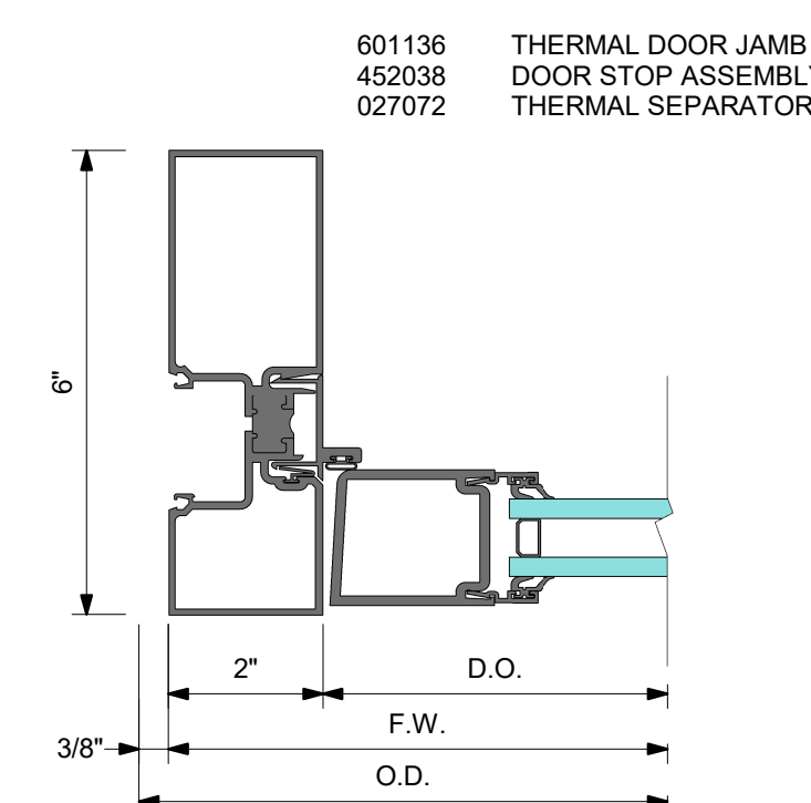
4 DETAIL 4 DOOR JAMB
