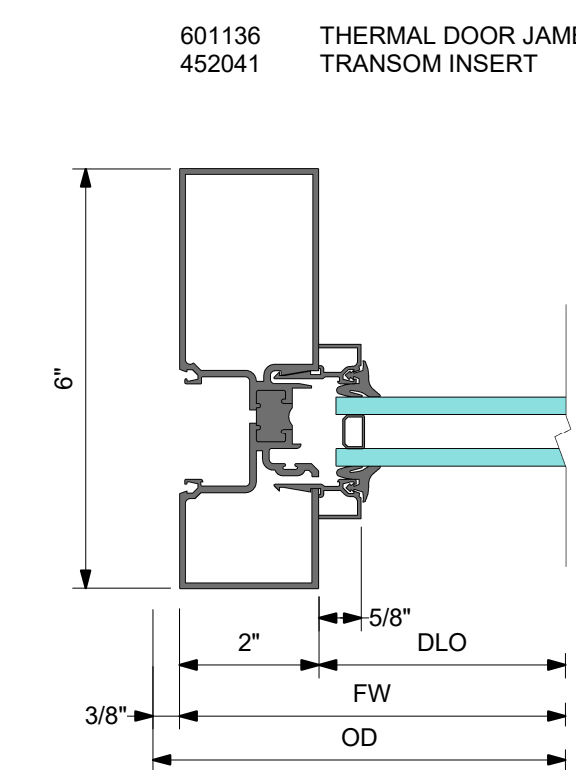
4A DETAIL 4A TRANSOM JAMB
