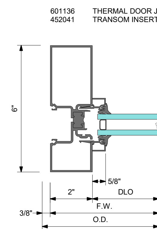
4A DETAIL 4A TRANSOM JAMB
