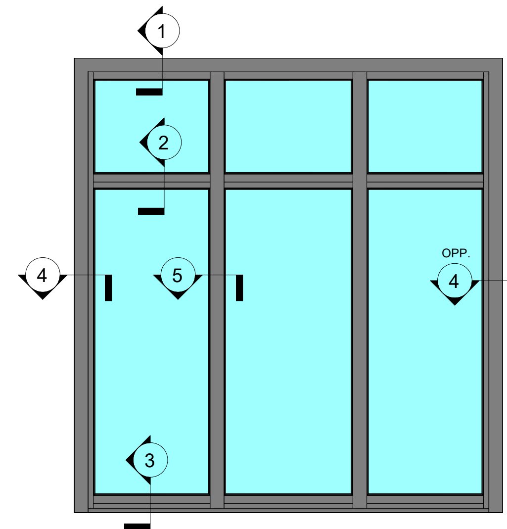
ELEVATION
