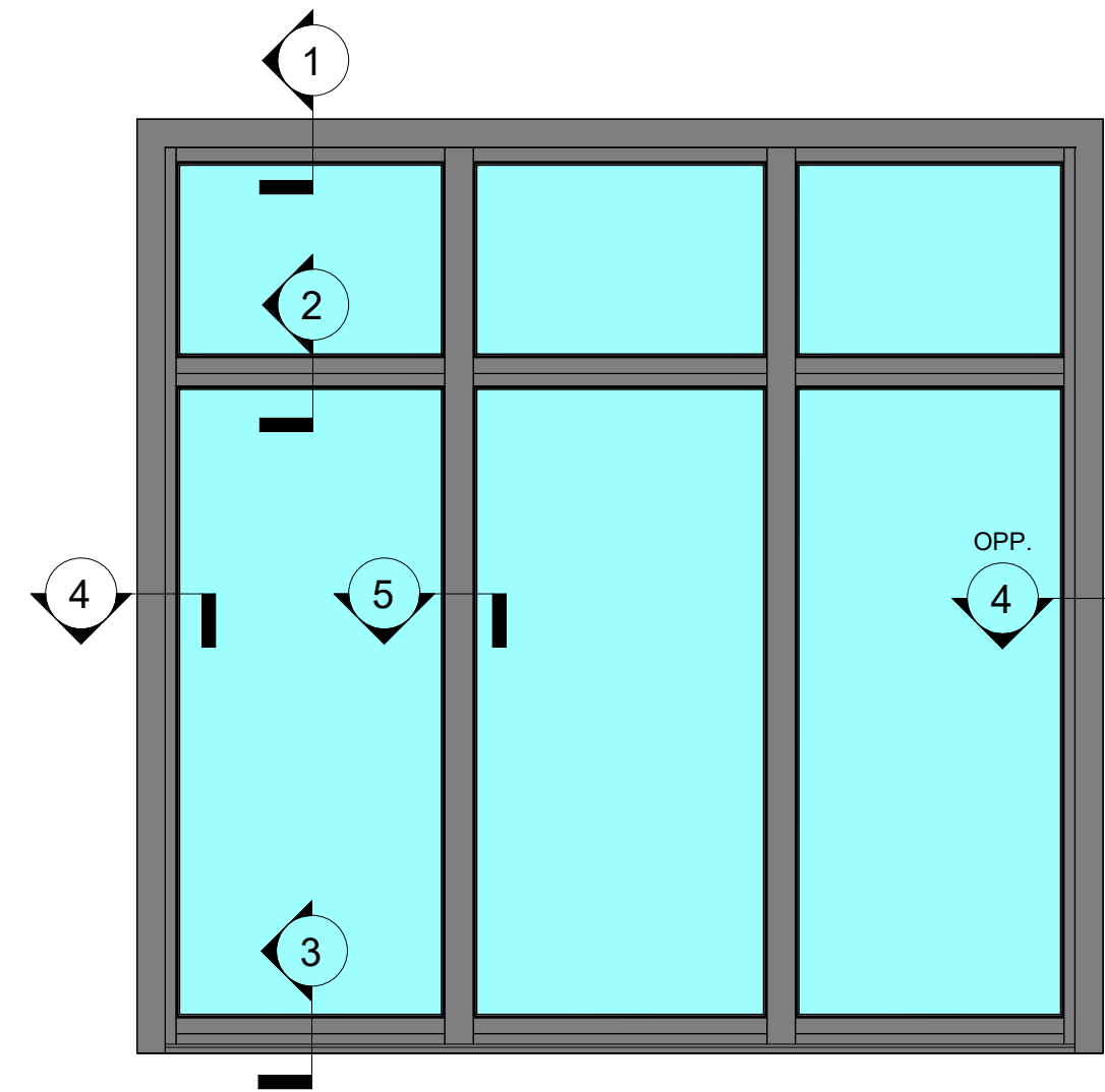
ELEVATION
