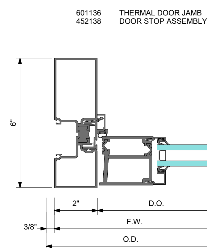
4 DETAIL 4 DOOR JAMB
